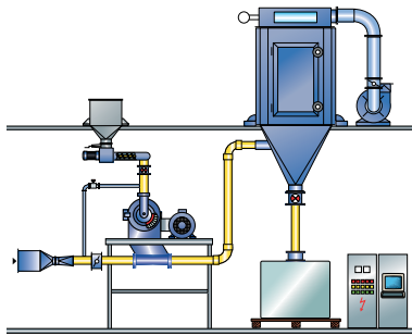
سیستم وکیوم / انتقال پنوماتیک
