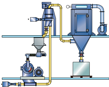
سیستم جداسازی مدار بسته
