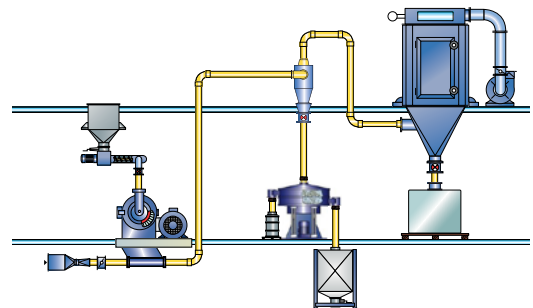
سیستم جداسازی مدار باز
